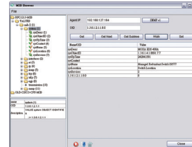
MIB Browser
